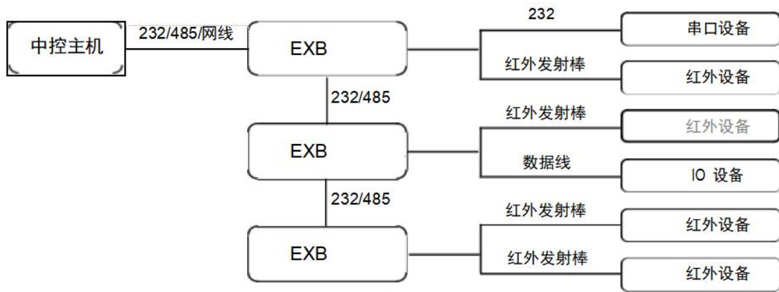
典型设备连接图
